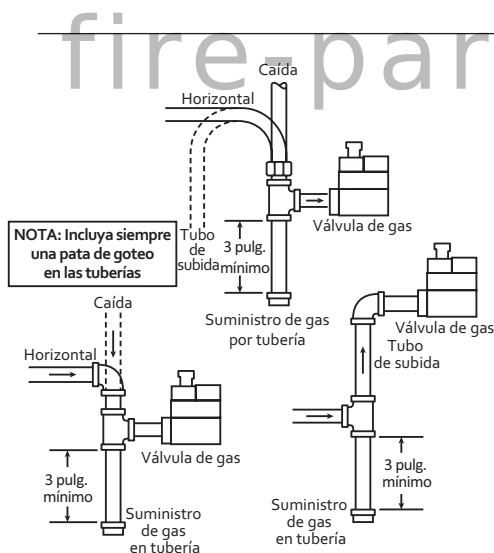
Figura 3. Tubería de válvula de gas típica
