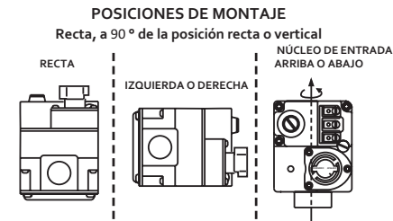
Figura 1. Posiciones de montaje de la válvula de gas
