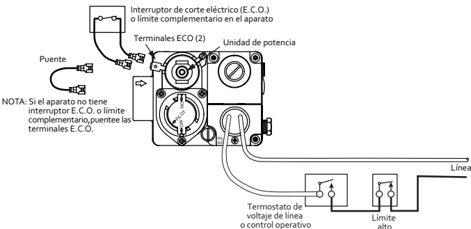
Figura 7. Cableado para el 36C03A (120 voltios)
